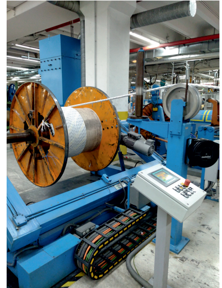
Bild 2. Bewährter Kabelaufwickler mit neuer Sicherheitstechnik © Euchner
